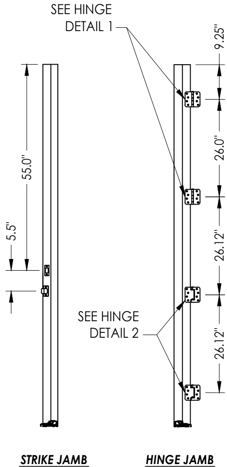
STRIKE JAMB
